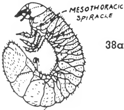
Fig. 92. Anomala kansanos Hayes & McColloch.
